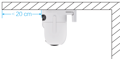
Fig. 2 Montagem na parede
